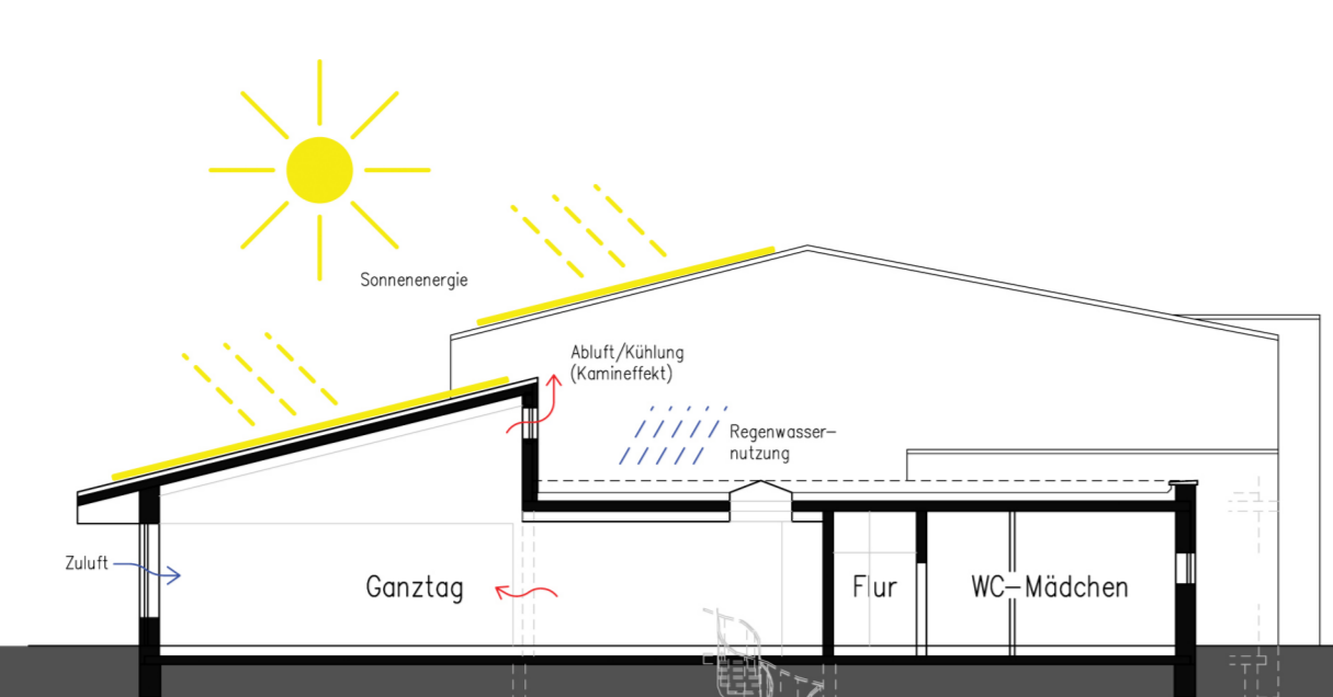
Gebäudeschnitt B-B
