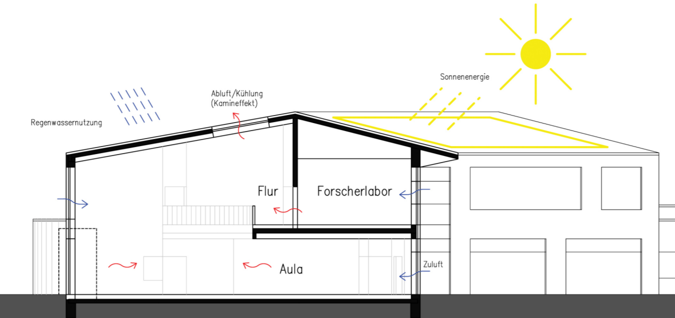
Gebäudeschnitt C-C
