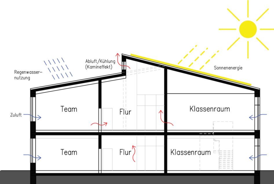
Gebäudeschnitt A-A
